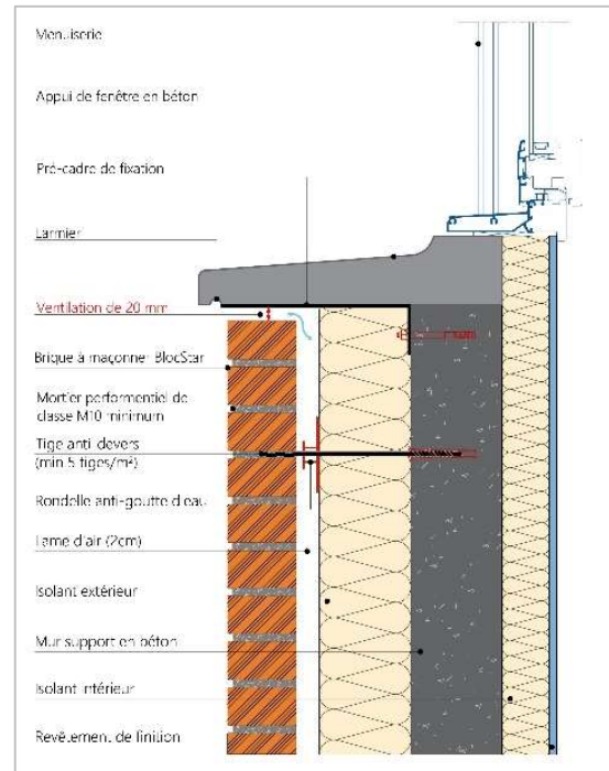
Fig. 4 - Détail d'appui de baie en béton
