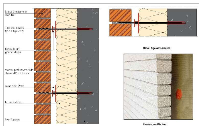
Fig. 2- Détail d'un double mur avec isolation par l'extérieur
