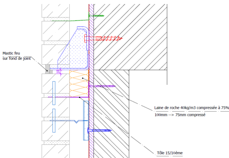
Figure 11 – Protection de la console en situation d'incendie – solution privilégiée
