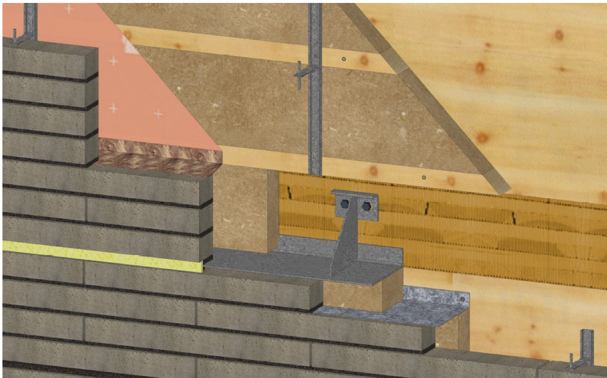
Figure 4 – Cas d'un mur porteur en panneau structural massif bois (p.ex. Structure CLT) – Ecran thermique laine de roche
