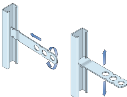
Figure 6 – Principe du rail ANCON 25/14 et de l'attache à blocage de forme ANCON YD25 ou YP25
