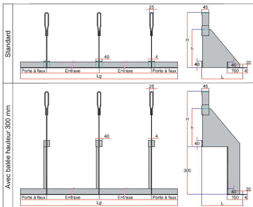
Figure 9 – Consoles ETANCO LR BRICK (support béton) pour nu de 160 à 260 mm (avec ou sans batée)
