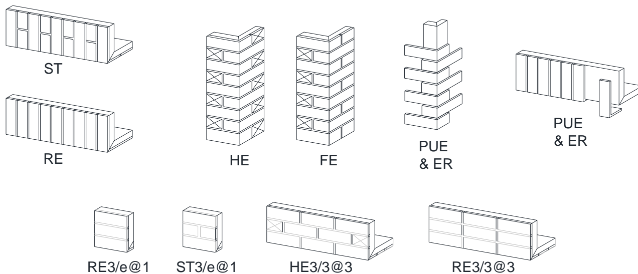
Figure 3 – Eléments d'angle
