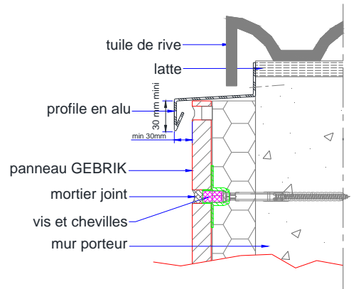
Figure 13 – rénovation bavette protectrice
