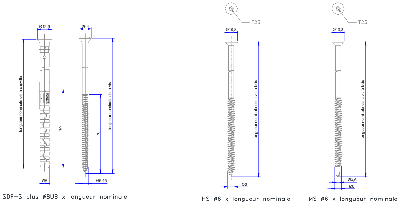
Figure 4 – Fixation des éléments
