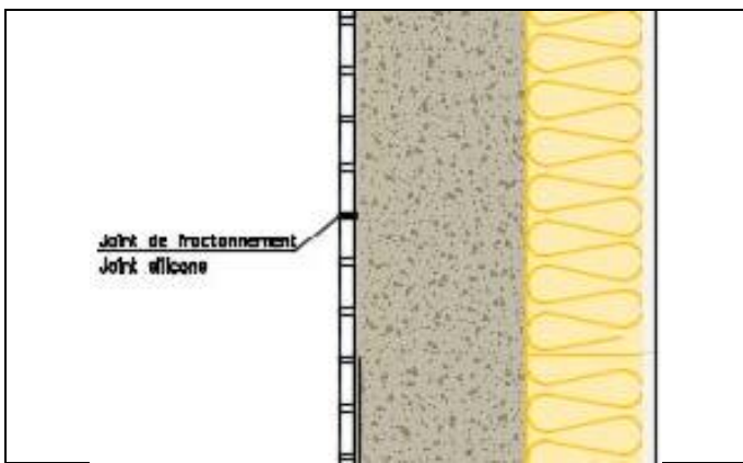
Figure 7 – Joint de fractionnement horizontal
