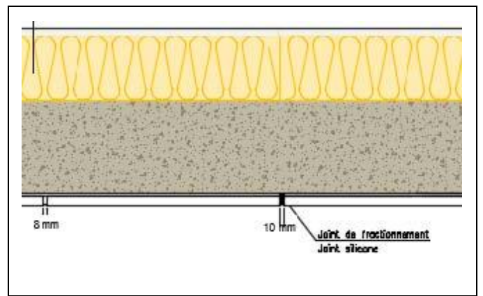
Figure 8 – Joint de fractionnement horizontal
