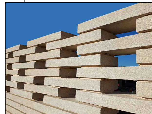
Moucharabieh non contreventé en briques Am 180 (18cm)
