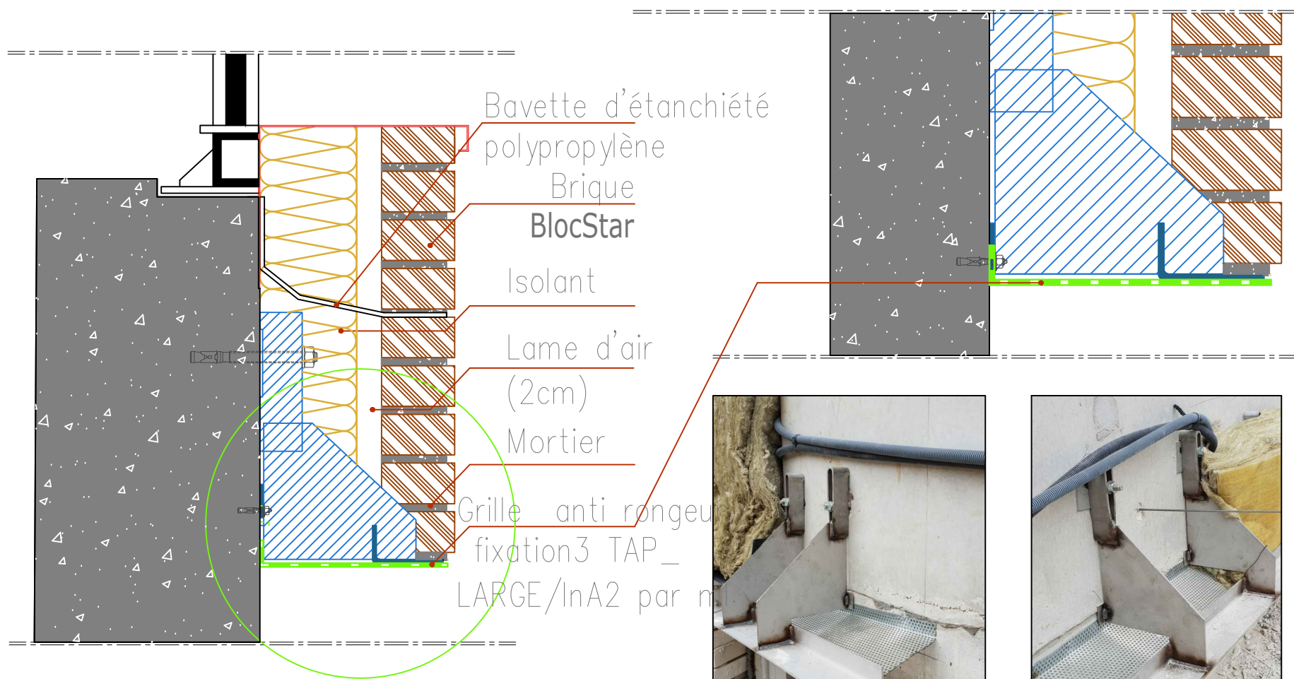
Coupe verticale
