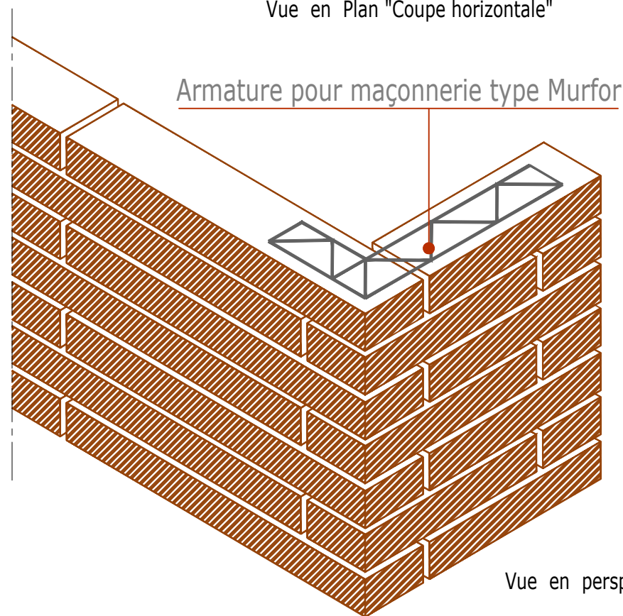
Armature pour maçonnerie type Murfor
